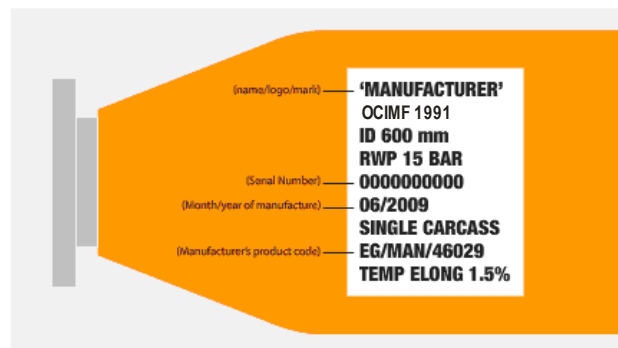
Εικόνα: Προβλεπόμενη σήμανση των υποβρύχιων αγωγών
